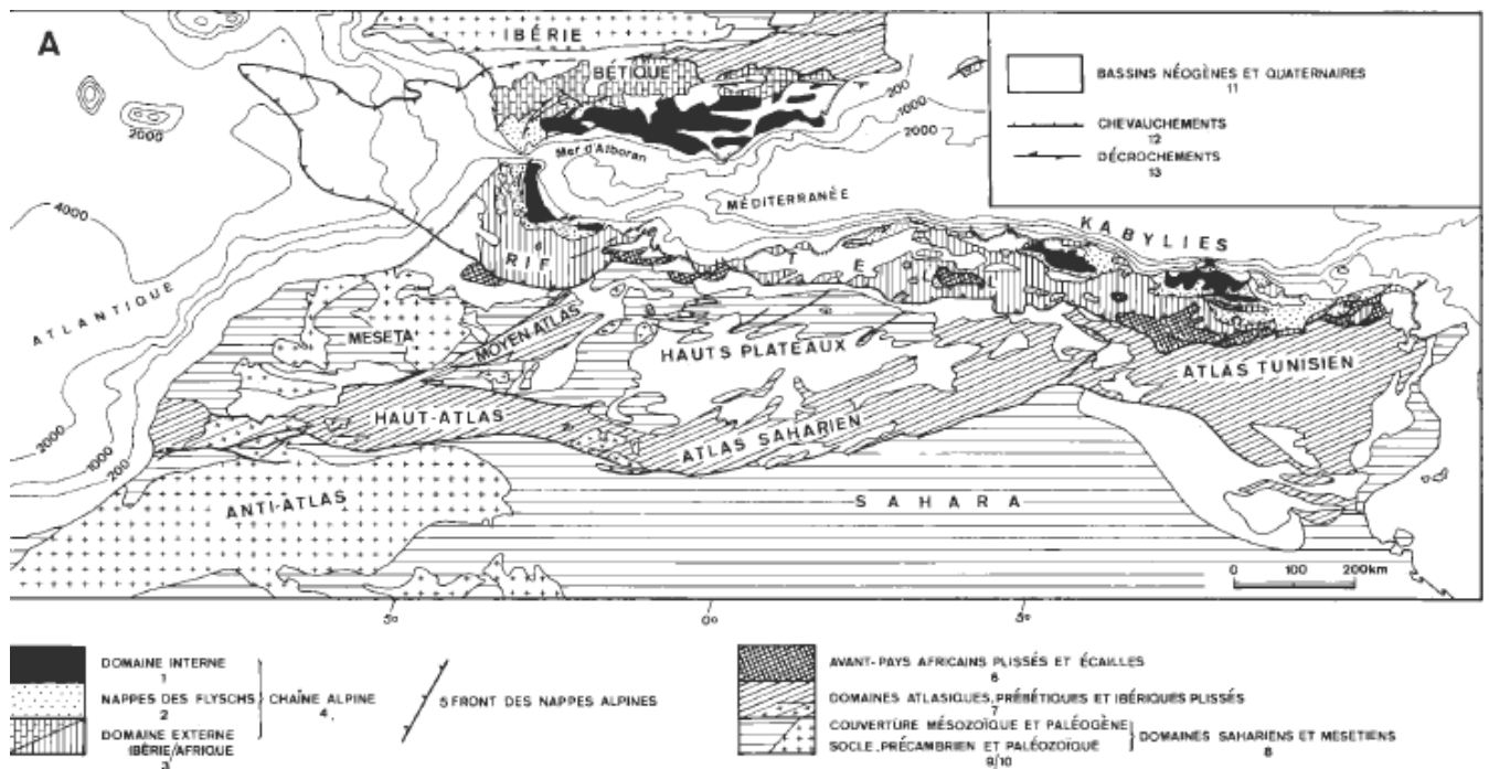
Fig 12. : Cadre structural africain et ibérique de la chaîne tello-rifaine (Wildi W.1983)
