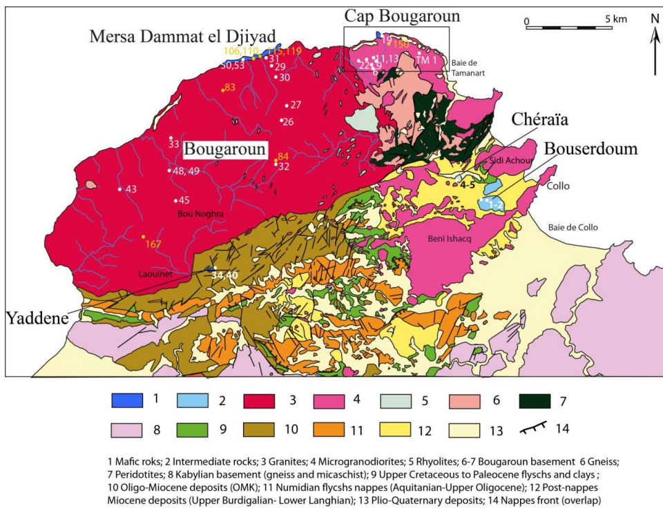
Fig.15- Carte géologique du massif de Bougaroun
