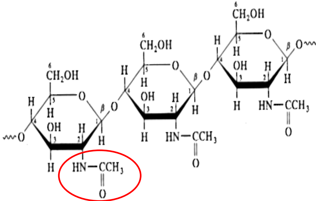
Groupe acétylamine
