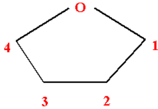
Furane réduit
