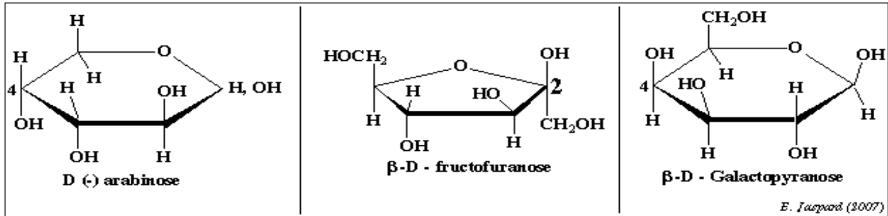
Furane réduit
