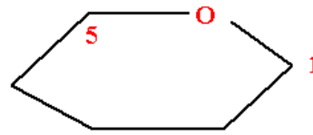
Pyrane réduit
