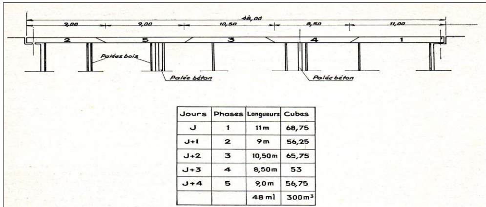
Fig.4 Phases de coulage d'un pont S.N.C.F Société Nationale des Chemins de Fer française.
