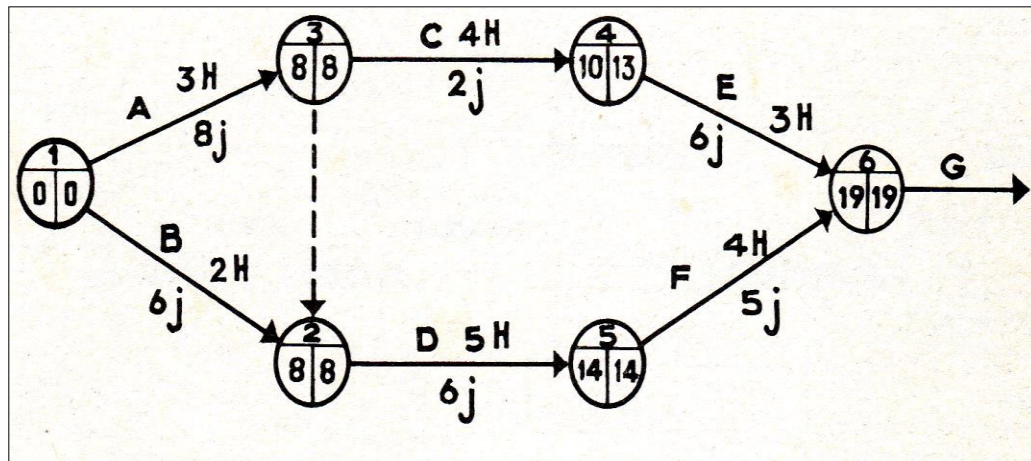
Fig.1 Type graphe potentiels – Etapes (ou méthode P.E.R.T).
