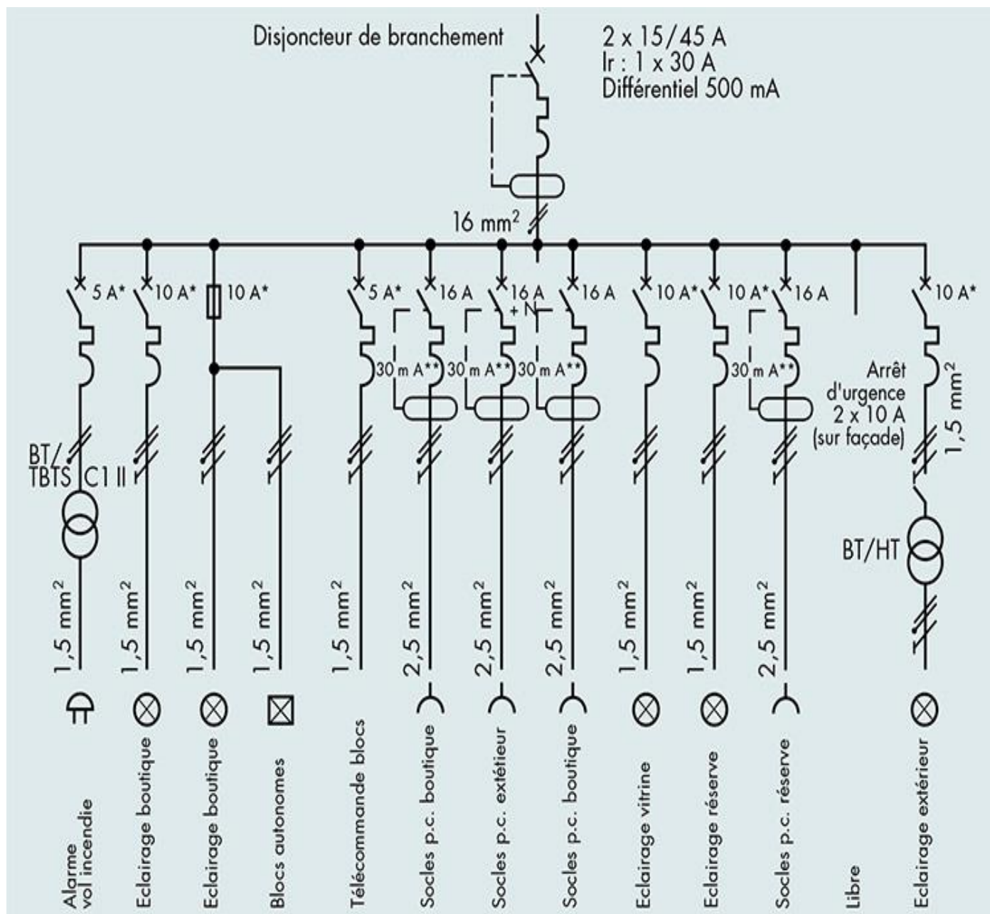
Installation électrique d'un local industriel
