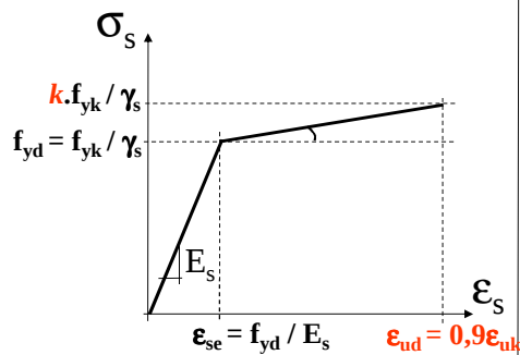
Diagramme à palier incliné (pour aciers A et B)
